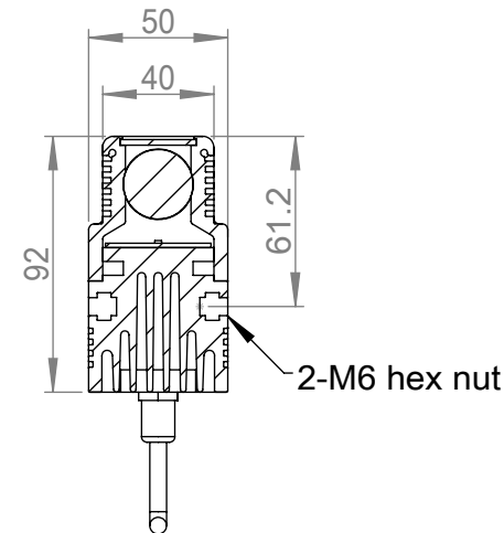
剖面 A-A
