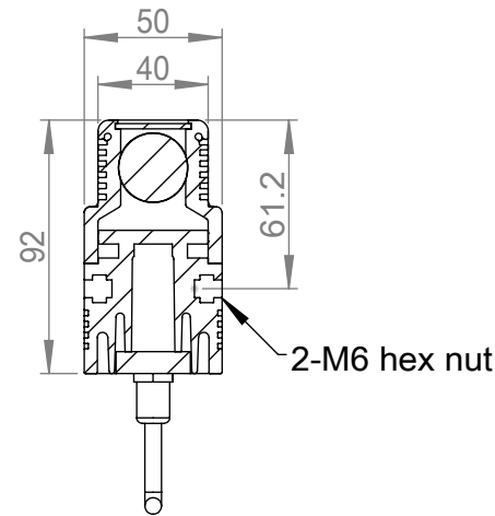
剖面 A-A
