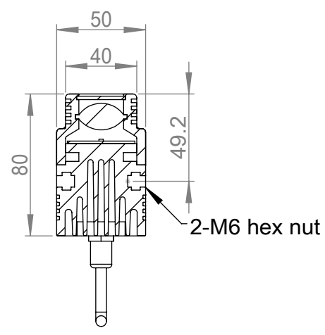
剖面 A-A
