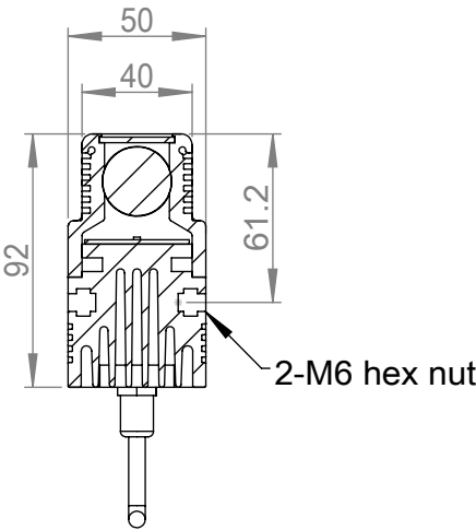
剖面 A-A
