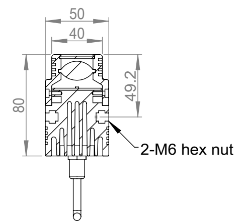
剖面 A-A
