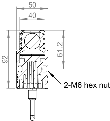
剖面 A-A
