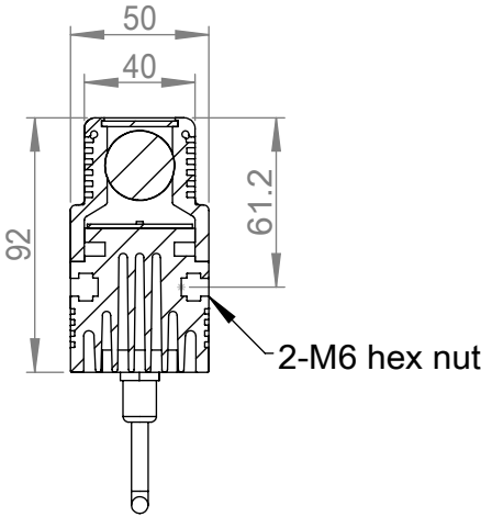
剖面 A-A
