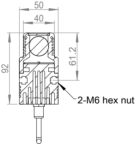
剖面 A-A
