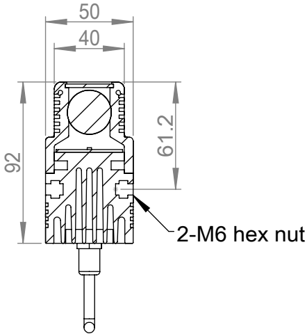
剖面 A-A
