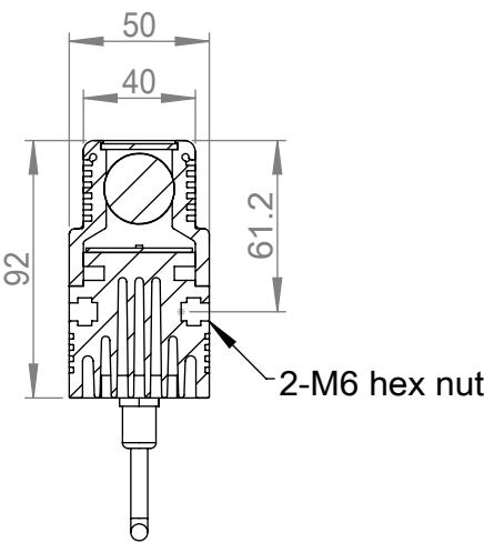
剖面 A-A
