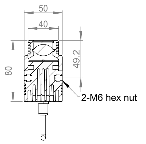
剖面 A-A
